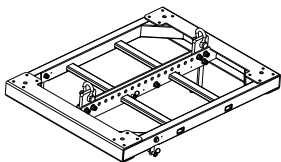
① IH-2810ZL 阵列吊架
